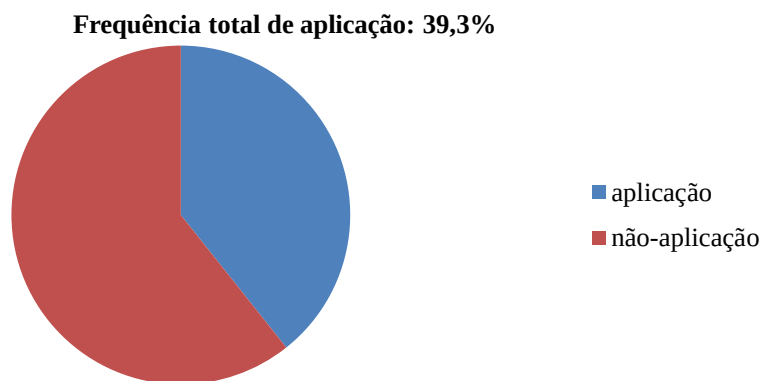
Gráfico 1 – Frequência total de aplicação de vibrante simples em Antônio Prado
