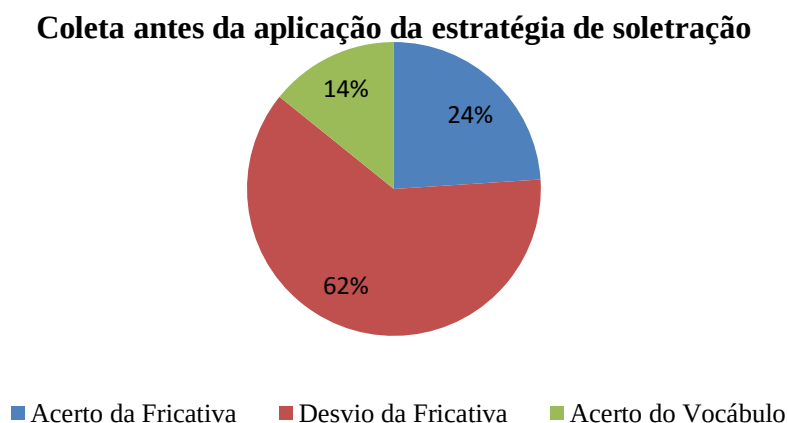
Figura 3 – Percentual de acertos e de desvios da fricativa /s/ e /z/ e do vocábulo todo antes da aplicação da estratégia de soletração
