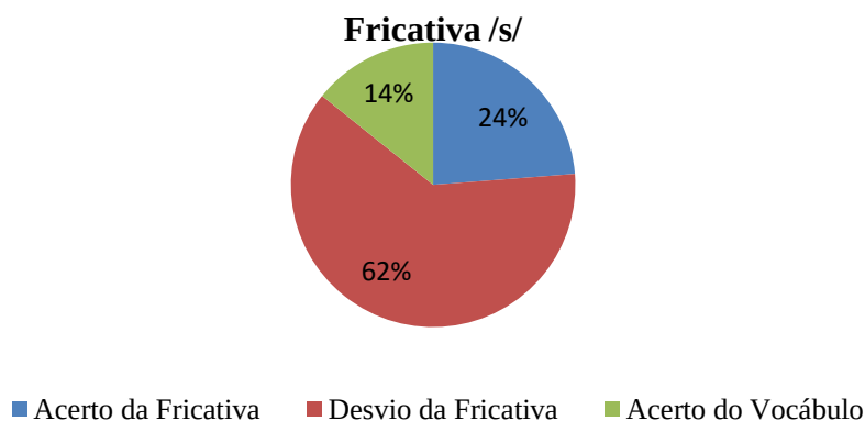
Figura 1 – Percentual de acerto e desvio da fricativa /s/ e de acerto do vocábulo todo
