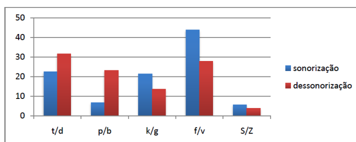
Gráfico 1: Distribuição dos erros por tipo de consoante e processo
