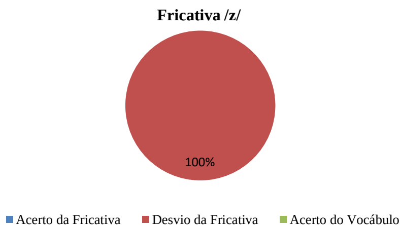
Figura 2 - Percentual de acerto e desvio da fricativa /z/ e acerto do vocábulo todo
