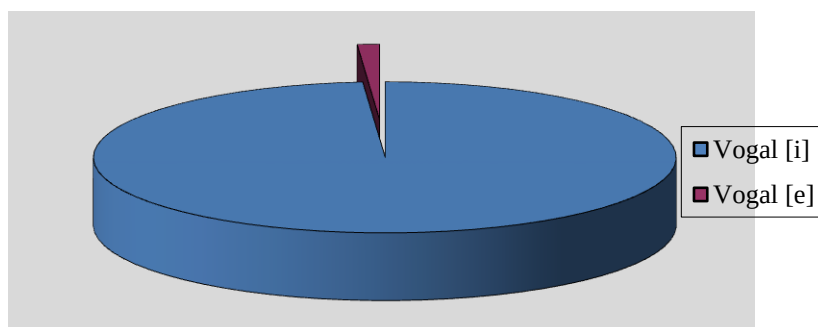
Gráfico 1 – Produções de epêntese com as vogais [i] e [e]
