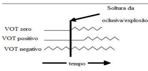
Figura 1: Tipos de VOT. 97
